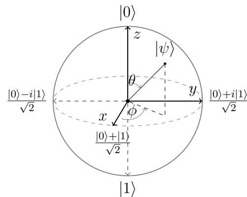
Figura 1 – Esfera de Bloch.
