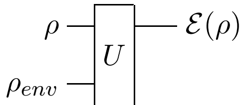
Figura 22 – Evolução com interferência do meio ambiente.
