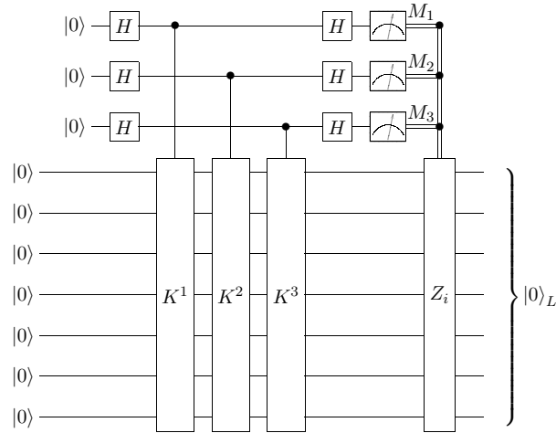
Figura 30 – Circuito para preparar |0\rangle^{\otimes 7} em |0\rangle_L do código de 7-qubits, após a medida das ancilas é aplicado uma porta Z no qubit i = 4M_1 + M_2 + 2M_3 - 1 .
