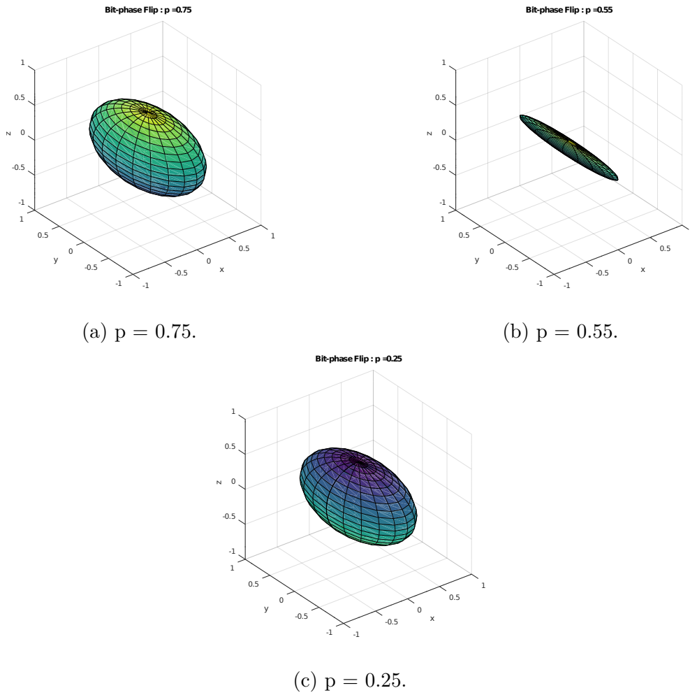
Figura 25 – Efeito do bit-phase flip na esfera de Bloch.
