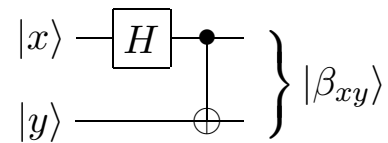
Figura 19 – Circuito de Bell.
