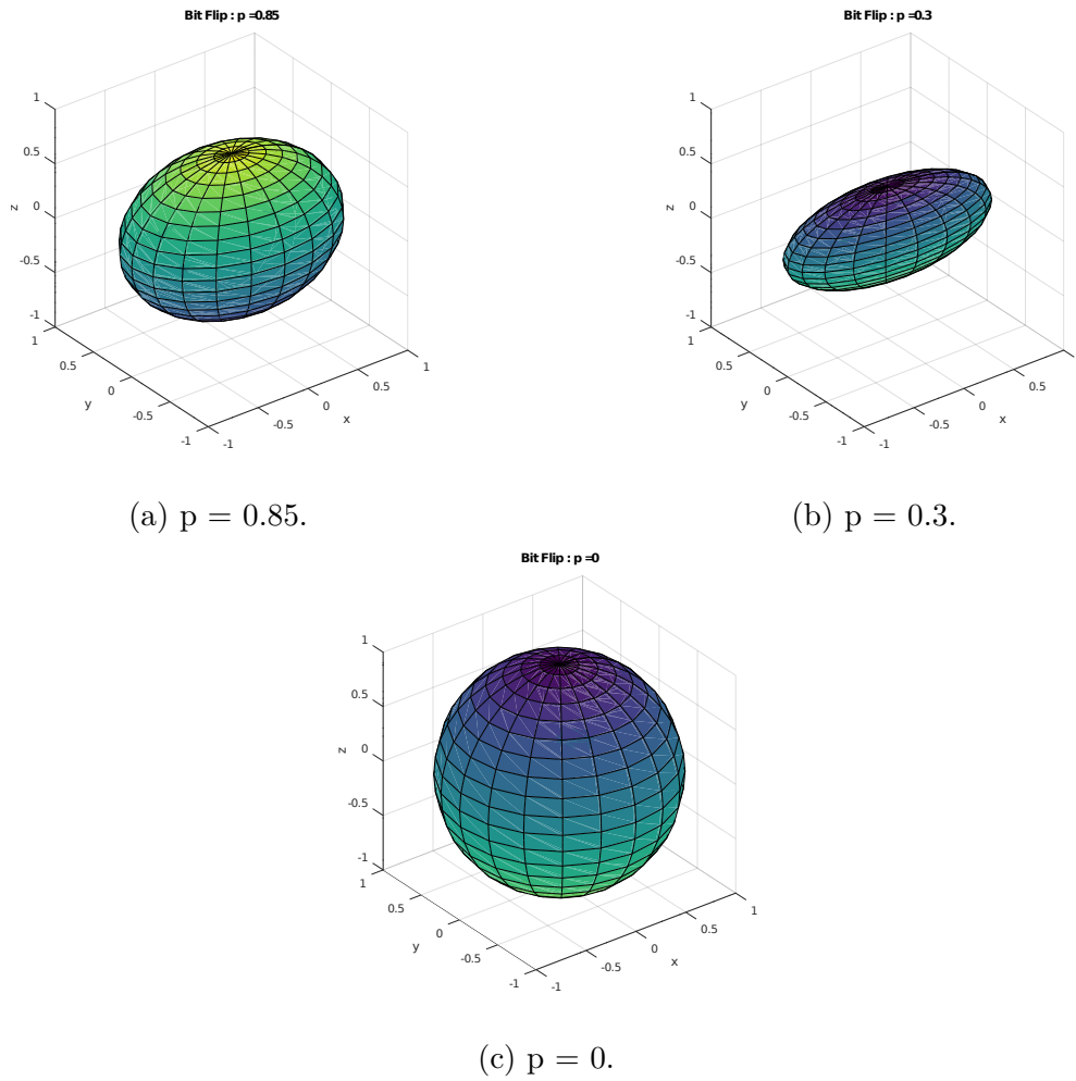
Figura 23 – Efeito do bit flip na esfera de Bloch.
