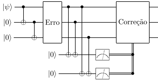
Figura 33 – Código de correção de bit flip .
