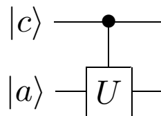
Figura 12 – A operao U_{c,a} |c\rangle |a\rangle s3 ser4 aplicada se |c\rangle = |1\rangle .
