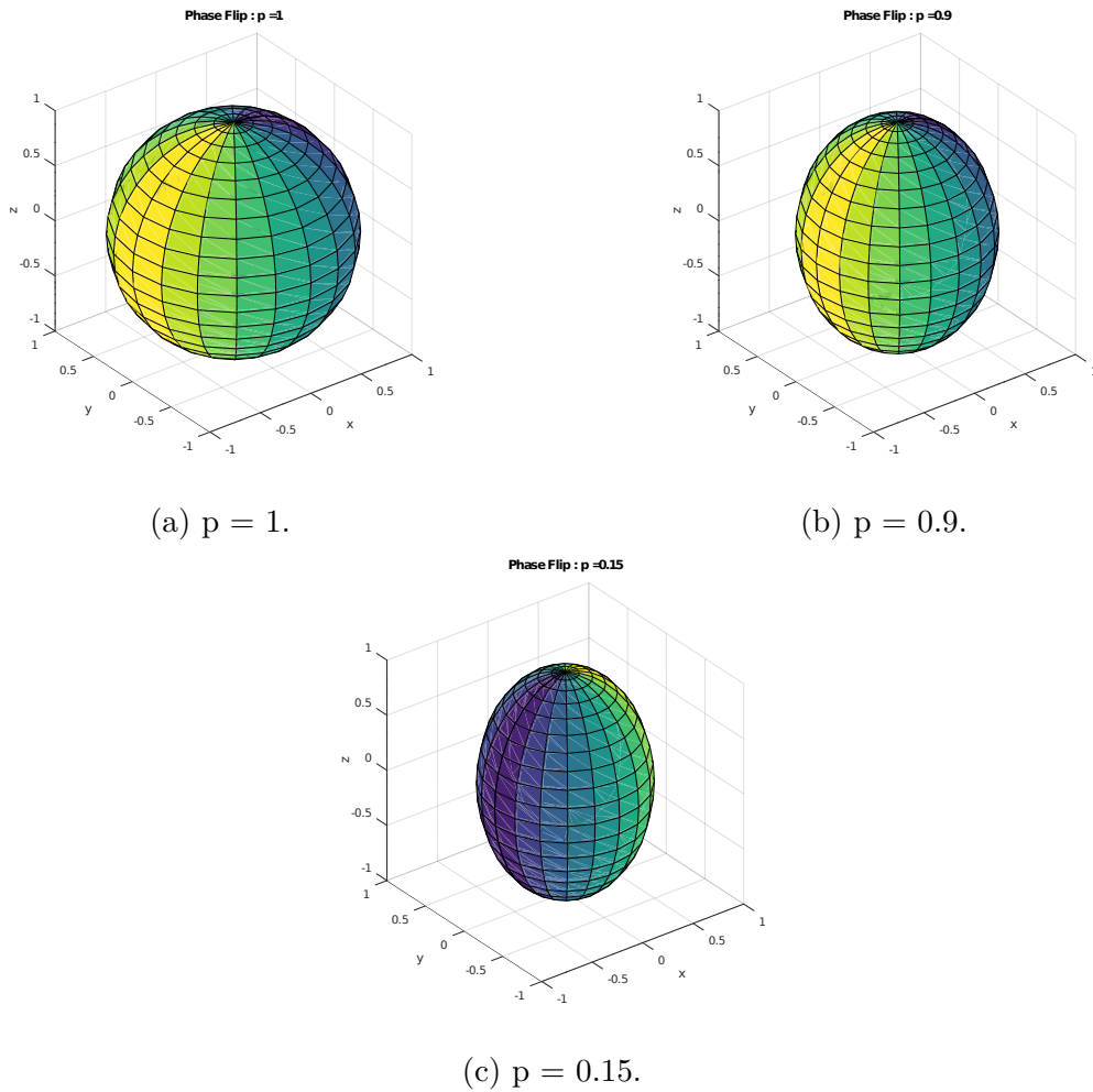
Figura 24 – Efeito do Phase flip na esfera de Bloch.
