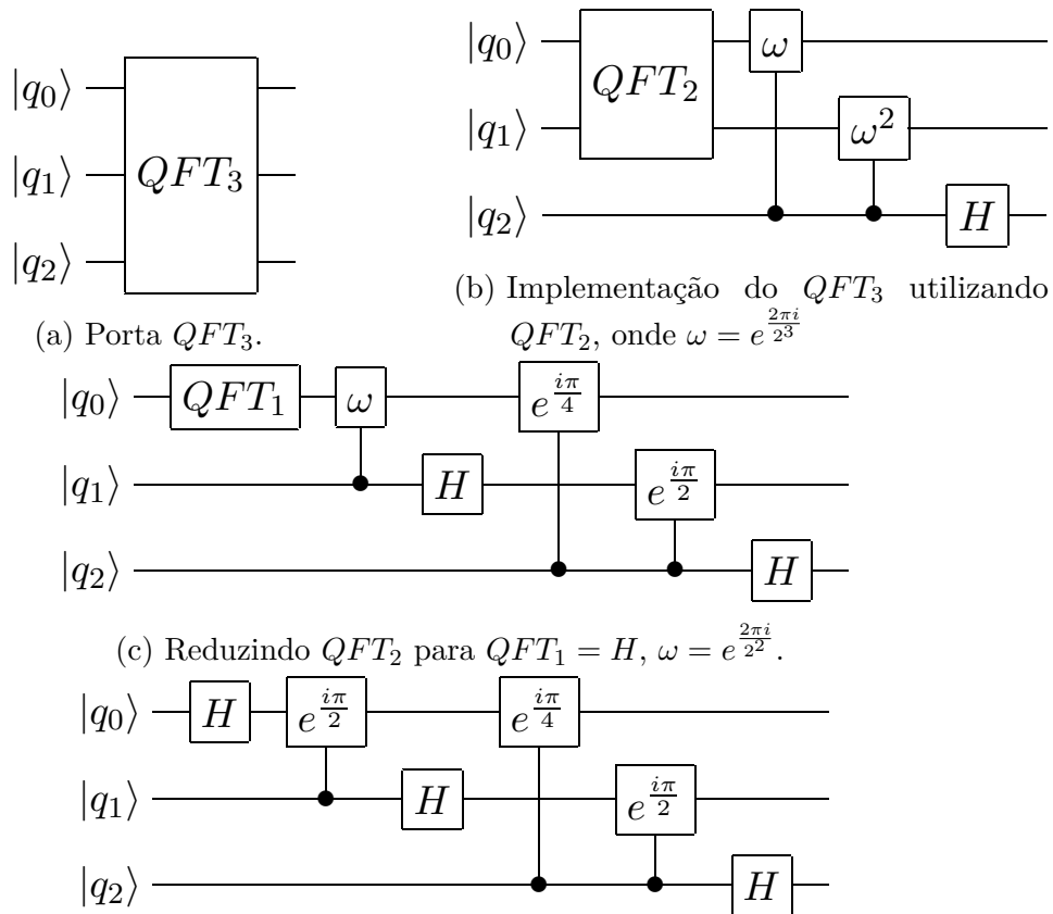
Figura 20 – Processo recursivo de criação do circuito que implementa QFT_3 .
