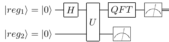
Figura 3. Circuito quântico utilizado para encontrar o período da função a^x \bmod n . Os registradores quânticos |reg_1\rangle e |reg_2\rangle devem ser compostos de \lceil \log_2(n+1) \rceil qubits. A porta lógica quântica U mapeia |x\rangle|0\rangle para |x\rangle|a^x \bmod n\rangle .
