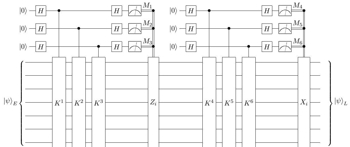
Figura 31 – A medida de síndrome para código de Steane é dividida em duas partes, onde, a primeira, identifica e corrige phase flip aplicando uma porta Z no qubit i = 4M_1 + M_2 + 2M_3 - 1 e, a segunda, identifica e corrige bit flip aplicando uma porta X no qubit i = 4M_4 + M_5 + 2M_6 - 1 .
