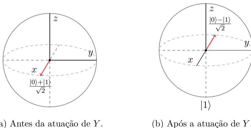
Figura 4 – Efeito da aplicação de Y .
