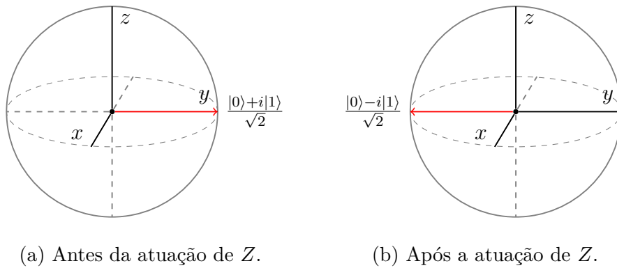
Figura 3 – Efeito da aplicação de Z .
