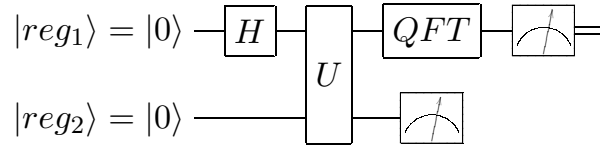
Figura 29 – Circuito quântico utilizado para encontrar o período da função a^x \pmod n . Os registradores quânticos |reg_1\rangle e |reg_2\rangle devem ser compostos de \lceil \log_2(n+1) \rceil qubits. A porta lógica quântica U mapeia |x\rangle|0\rangle para |x\rangle|a^x \pmod n\rangle .
