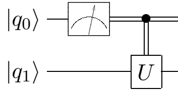
Figura 18 – A medida de |q_0\rangle é usada como controle para porta U .
