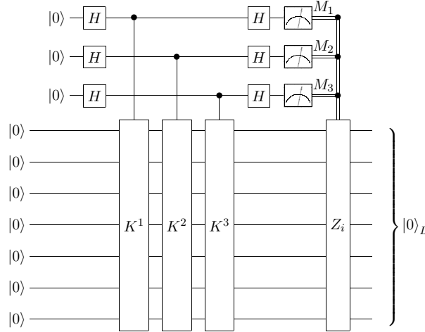
Figura 37 – Circuito para preparar |0\rangle^{\otimes 7} em |0\rangle_L do código de 7-qubits, após a medida das ancilas é aplicada uma porta Z no qubit i = 4M_1 + M_2 + 2M_3 - 1 .
