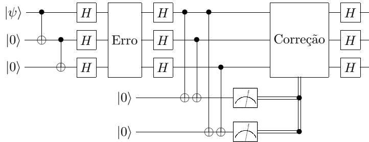
Figura 34 – Código de correção de phase flip .
