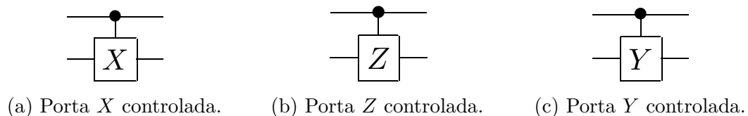
Figura 13 – Portas de Pauli controladas.
