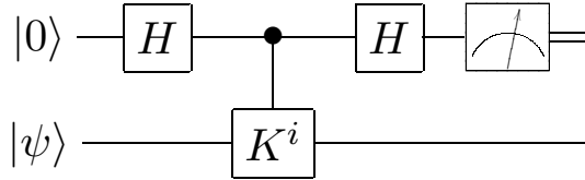
Figura 36 – Prepara |\psi\rangle como autovetor \pm 1 de K .
