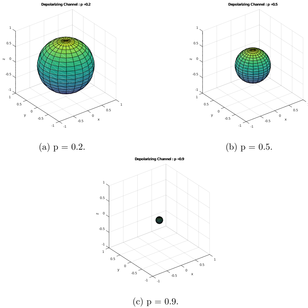
Figura 26 – Efeito do canal de despolarização na esfera de Bloch.
