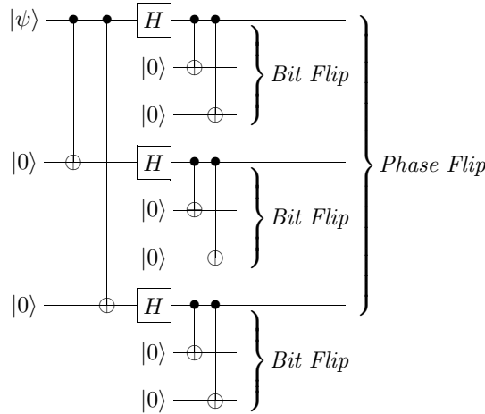
Figura 35 – Preparação do código de Shor.
