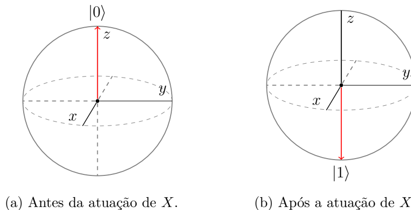
Figura 2 – Efeito da aplicação de X .
