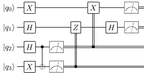
Figura 2. Exemplo de circuito quântico.
