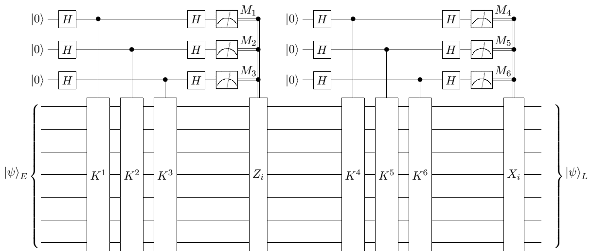
Figura 38 – A medida de síndrome para código de Steane é dividida em duas partes, onde, a primeira, identifica e corrige phase flip aplicando uma porta Z no qubit i = 4M_1 + M_2 + 2M_3 - 1 e, a segunda, identifica e corrige bit flip aplicando uma porta X no qubit i = 4M_4 + M_5 + 2M_6 - 1 .
