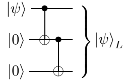
Figura 32 – Preparação do código repetição para bit flip .
