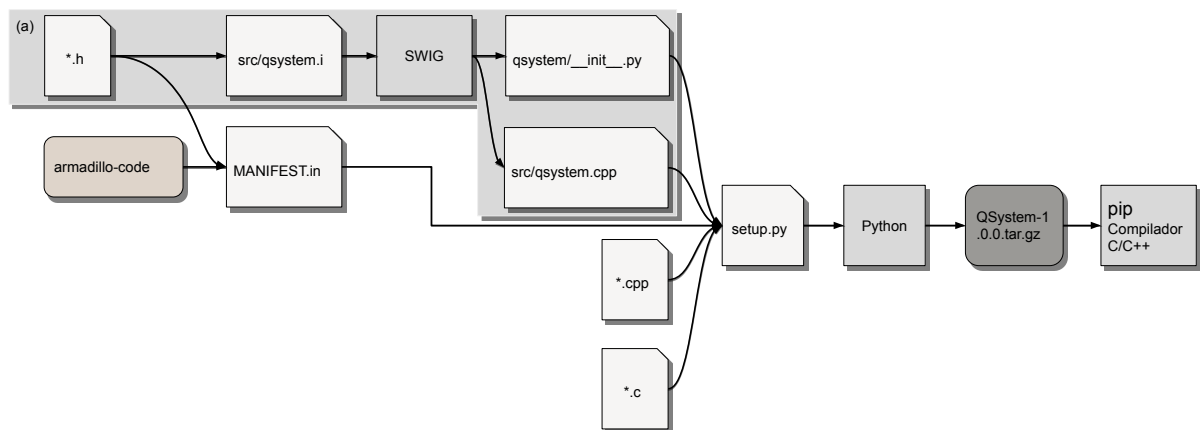
Figura 28 – Processo de criação do módulo QSystem. (a) interface C++/Python. Esse processo pode ser visto no Makefile disponível em D.2.
